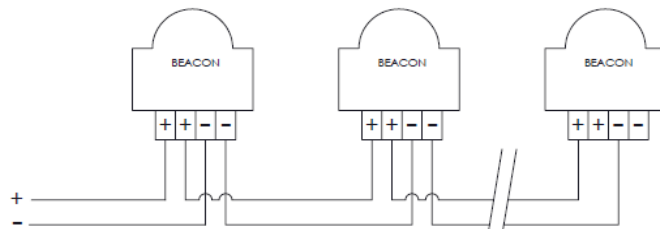
Abb. 7 DC Vereinfachtes Blockdiagramm (negative Ansteuerung)
