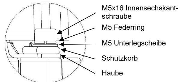
Abb. 13 Haube und Schutzkorb-Befestigung
