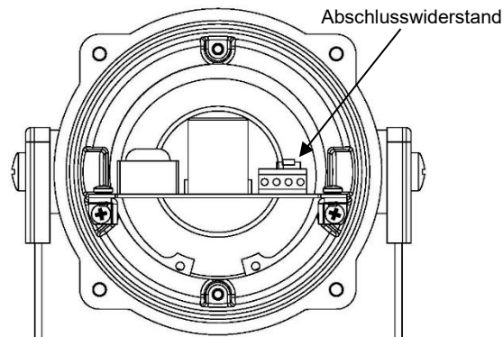
Abb. 9 Position des Abschlusswiderstandes
