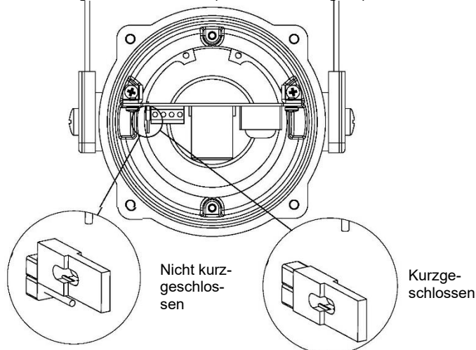
Abb. 10 Steckbrückenkonfiguration
