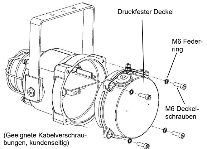
Abb. 2 Zugang zum explosionsgeschützten Gehäuse
