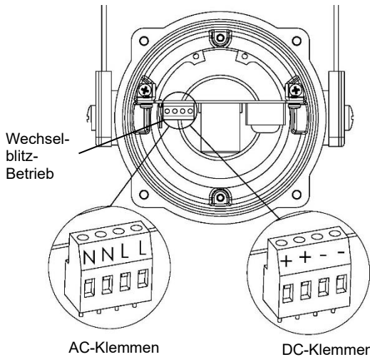
Abb. 4 Innenansicht der BExBGD-P 5-Joule-Leuchte
