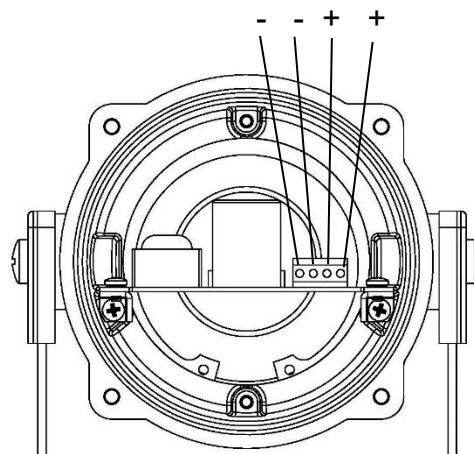
Abb. 8 DC-Klemmen
