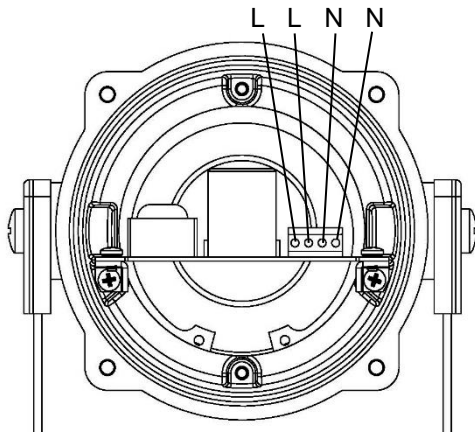
Abb. 6 AC-Klemmen
