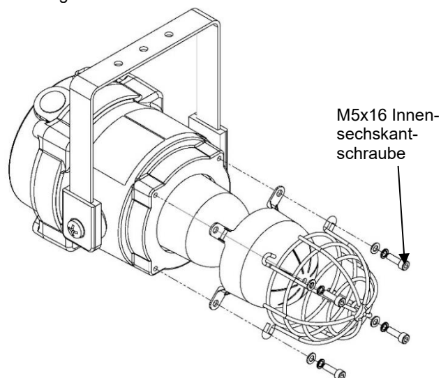
Abb. 11 Entfernen der Haube
