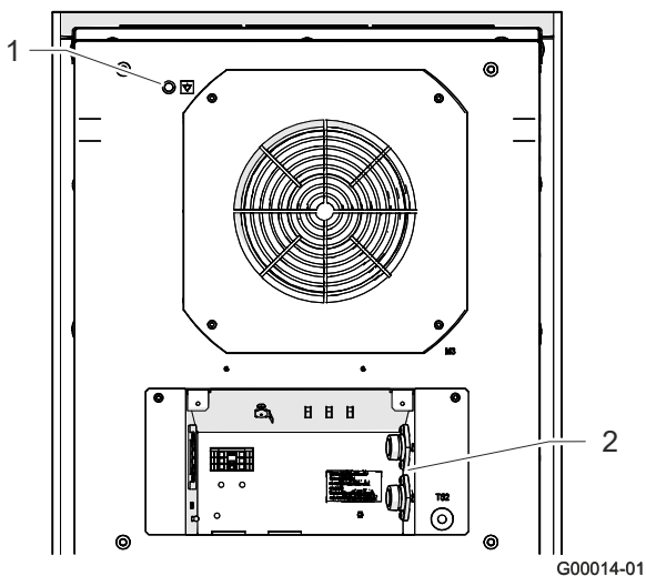
Abb. 21: Potentialausgleich / Sicherungen
