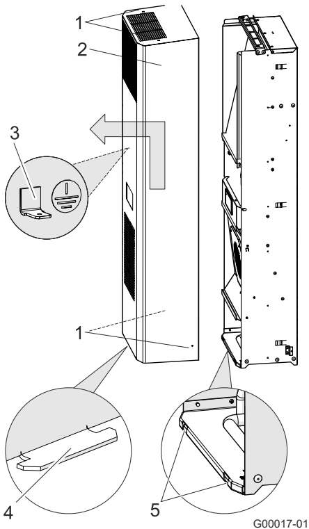
Abb. 24: Gerätehaube demontieren
