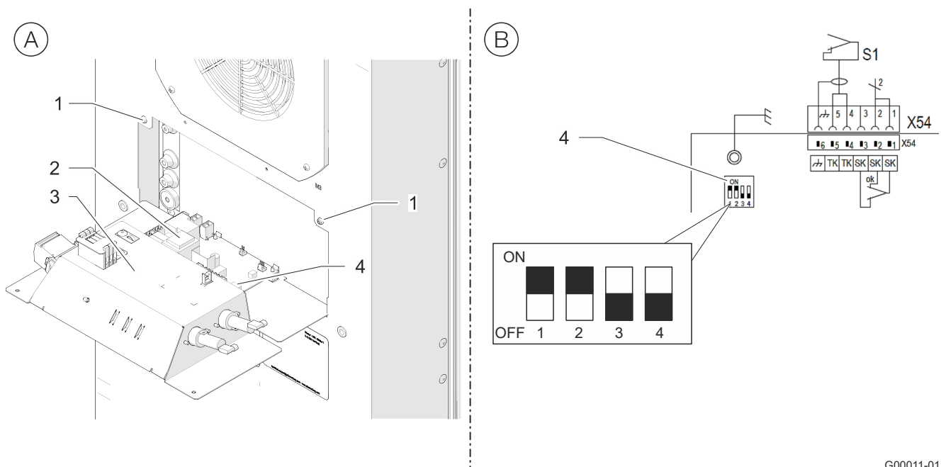
Fig. 16: réglage des commutateurs DIP
