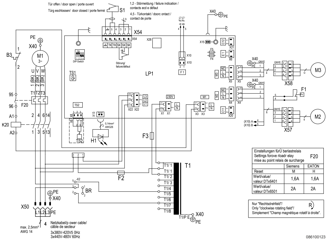
Fig. 14: Schema elettrico
