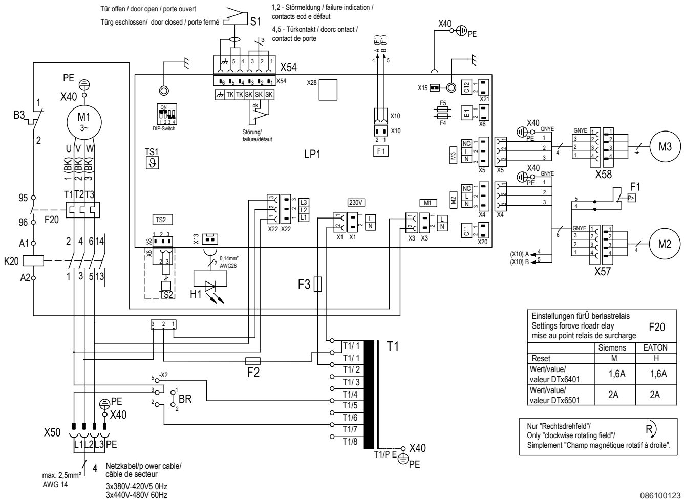
Abb. 14: Stromlaufplan
