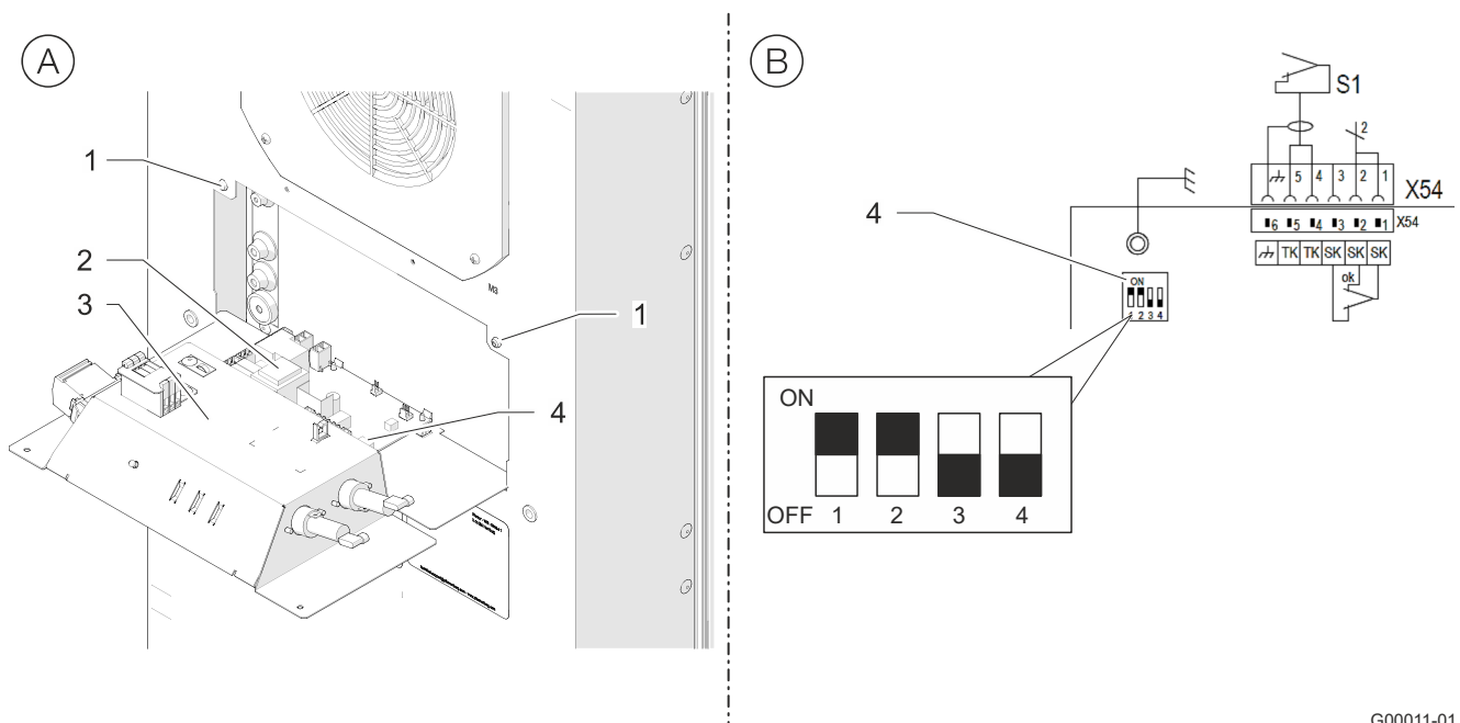
Fig. 16: Ajuste del interruptor DIP
