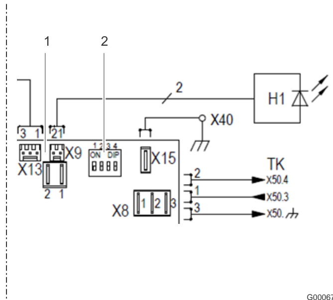
Commutateurs DIP
