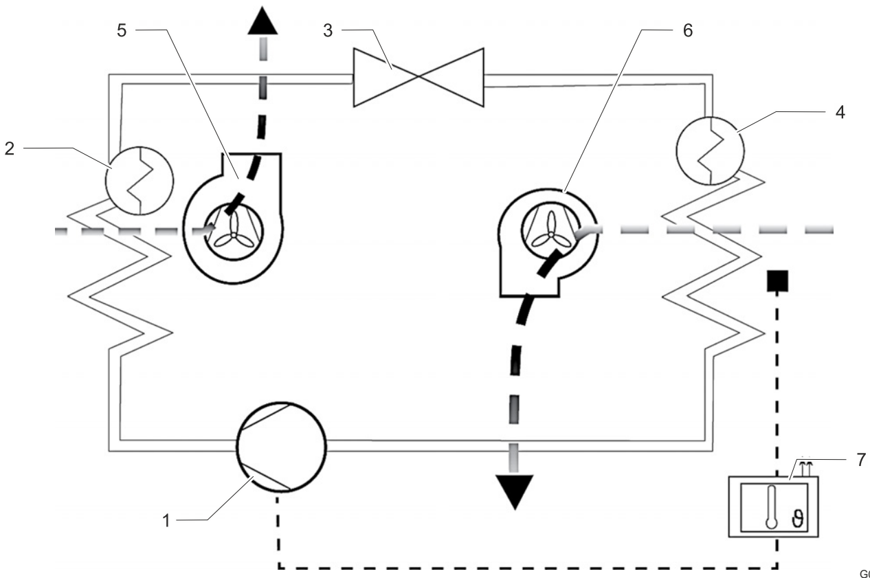
Рис. 8.: Холодильный контур
