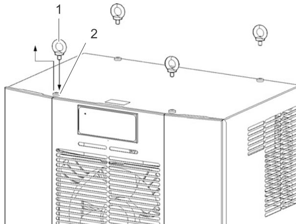
Рис. 12: Подъемные проушины М8 устройств охлаждения ДТТ
