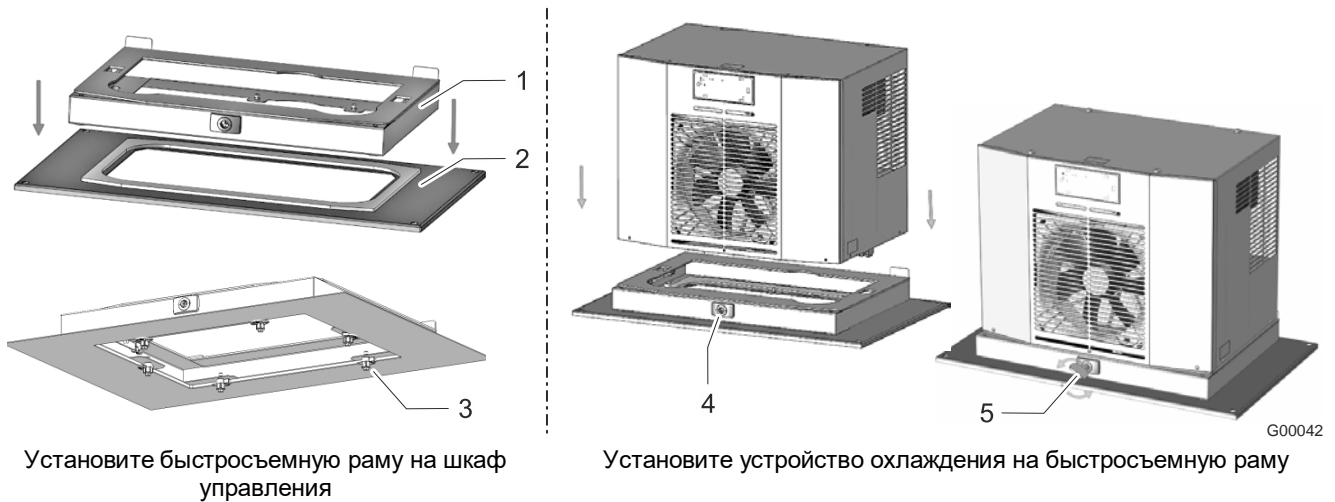
Рис. 19: Монтаж держателя
