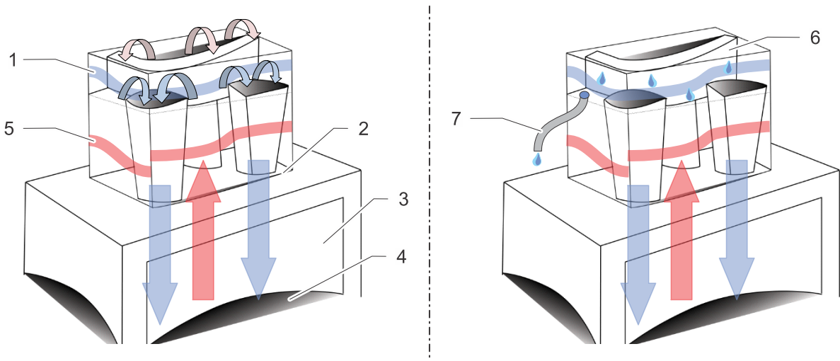
Расположение контуров охлаждения Рис. 9: Контур охлаждения и отвод конденсата
