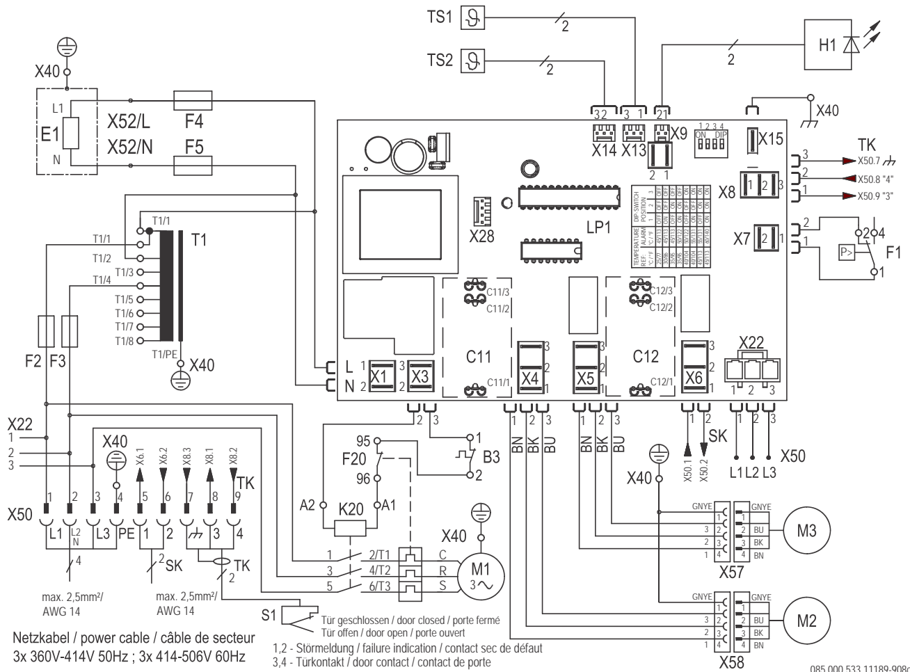
Fig. 20: Schema elettrico
