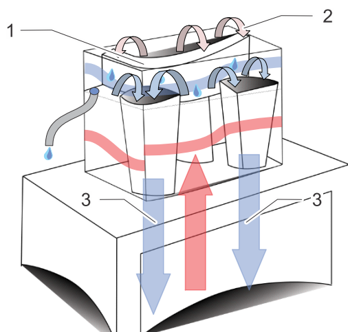
Funzione dell'evaporatore
