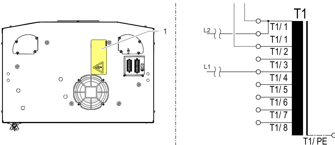
Werkseinstellungen Steuertransformator
