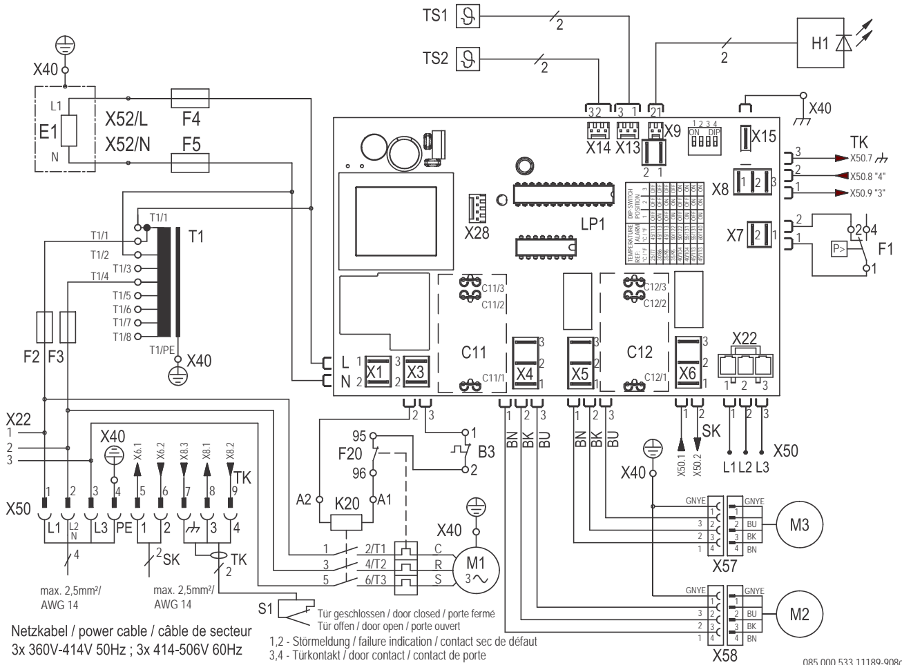
Abb. 20: Stromlaufplan
