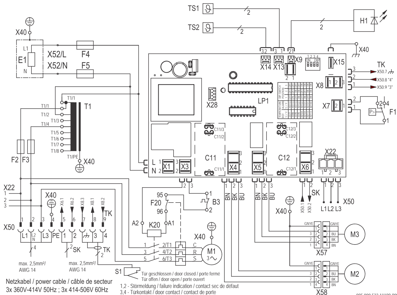
Fig. 20: Esquema eléctrico
