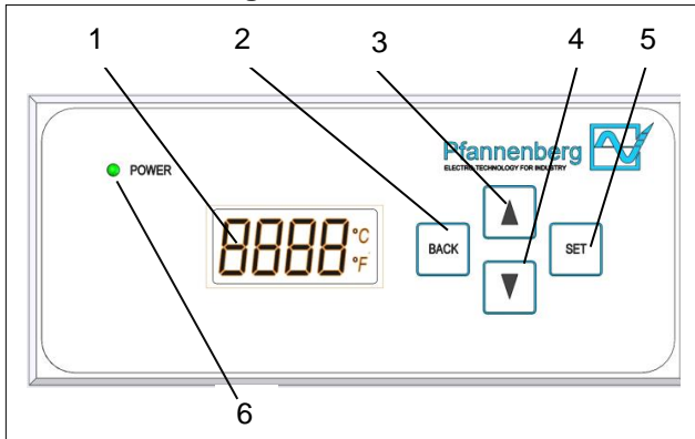
Abbildung 33 - Bedieneinheit (MC)
