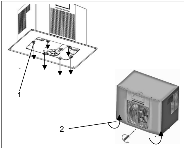
Figura 21: Separar la compuerta delantera
