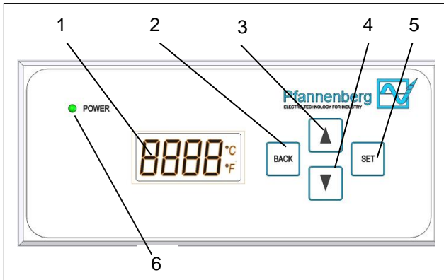
Illustration 33 - Unité de commande (MC)
