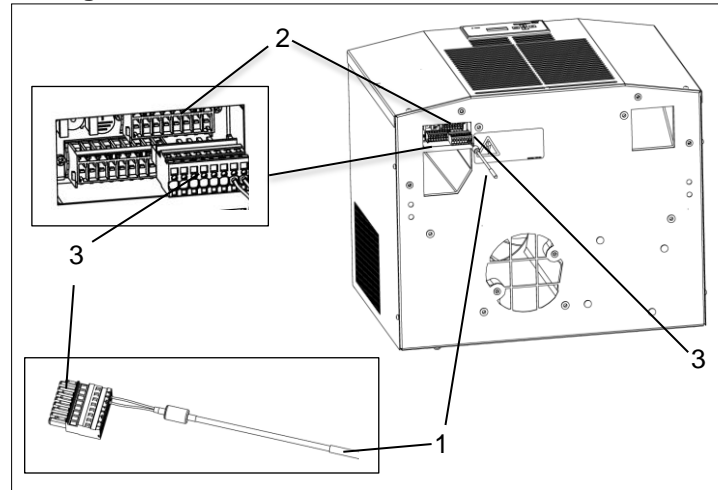
Illustration 14 – TS2- Capteur de température
