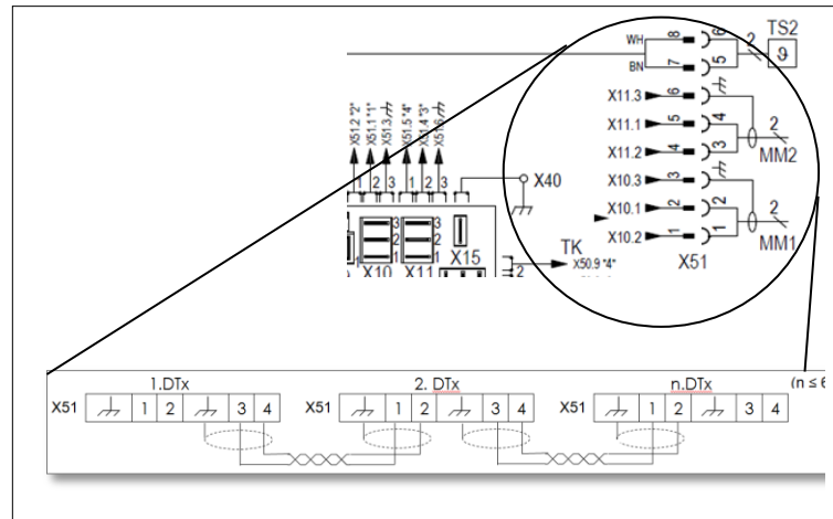
Abbildung 29 – Multimaster- Steuerung
