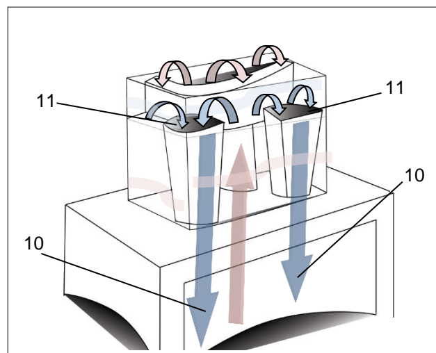
Рис. 13 - Воздушное охлаждение
