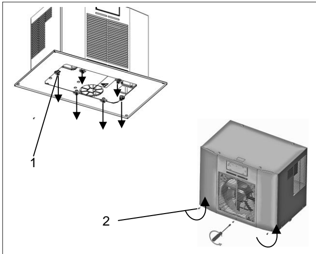
Immagine 22 – Svitare il coperchio frontale
