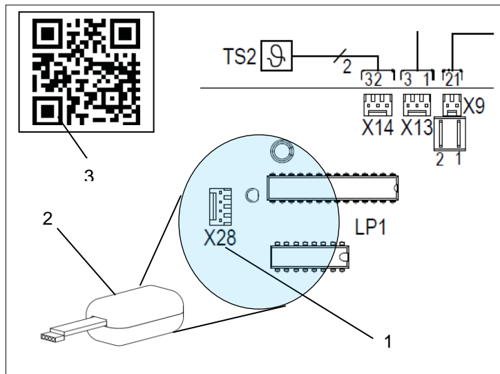
Abbildung 35 - Serviceschnittstelle
