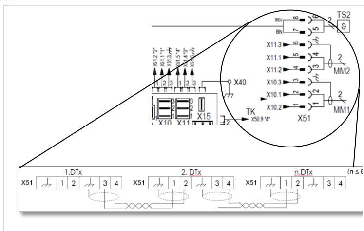
Immagine 15 – Dispositivo di controllo Multimaster
