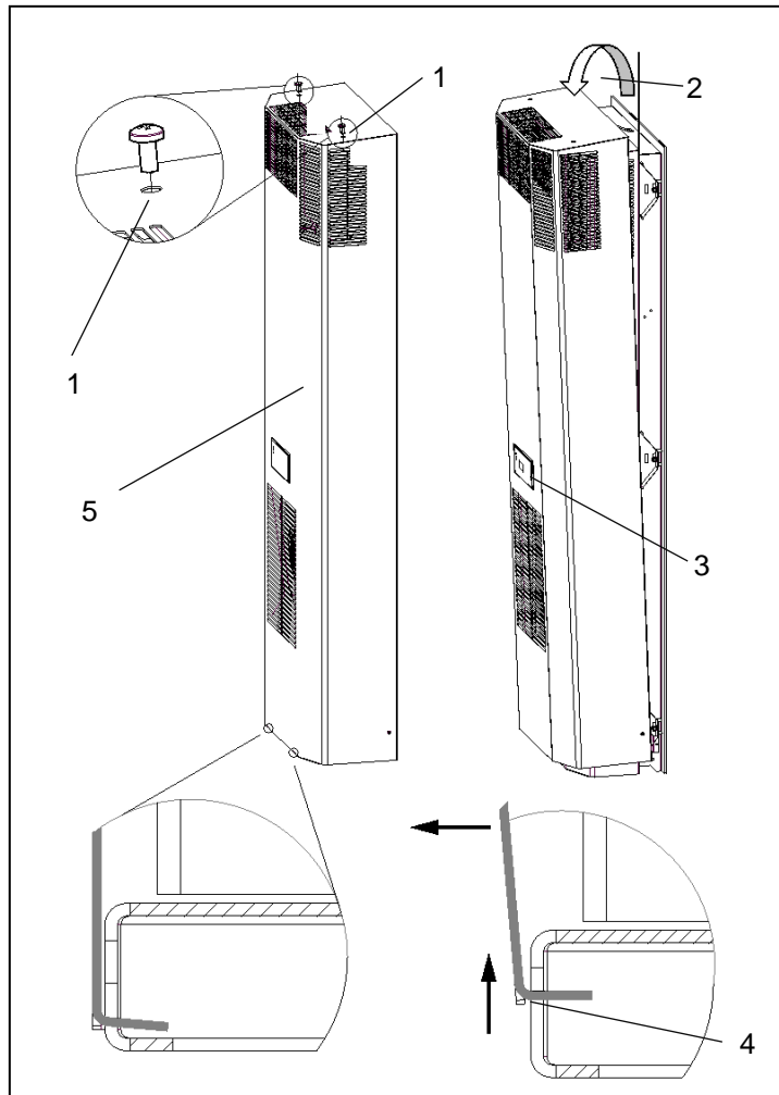
Figura 22: Desmontaje del protector de la unidad
