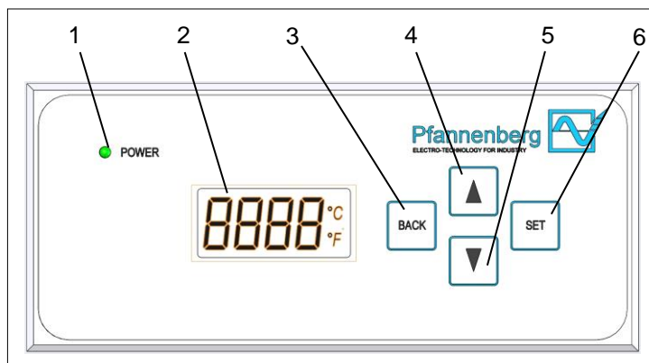
Abbildung 3 - Bedieneinheit Multi-Controller (MC)
