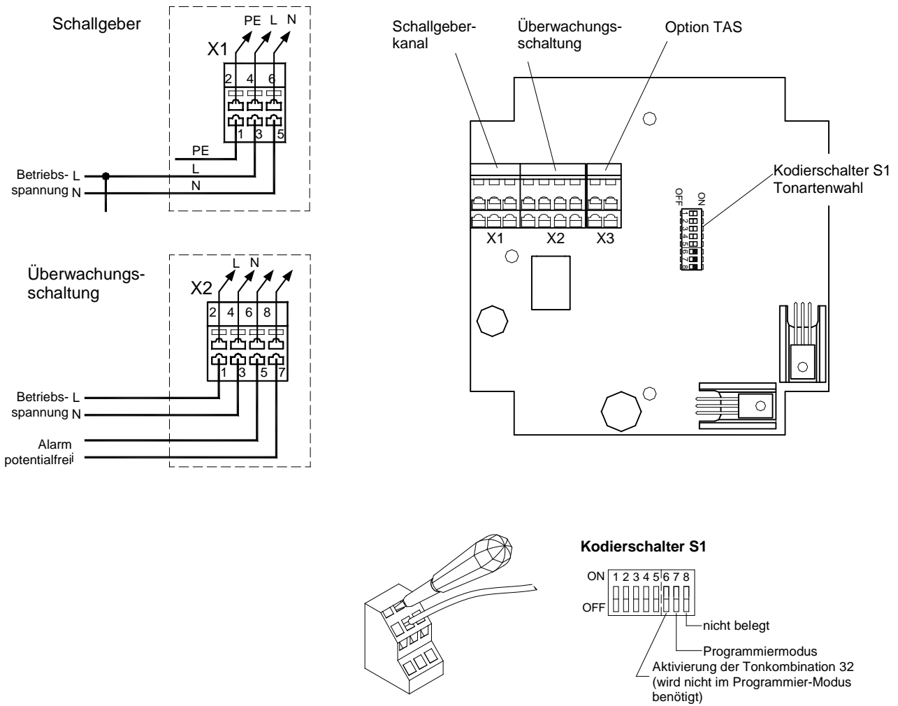
Abb. 10 Anschlussbelegung und Bedienelemente
